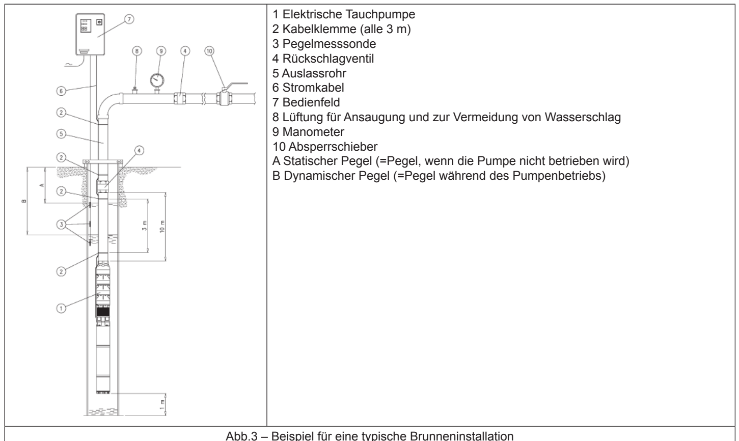
Abb.3 – Beispiel für eine typische Brunneninstallation
